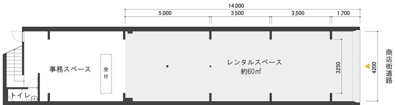
平面図
